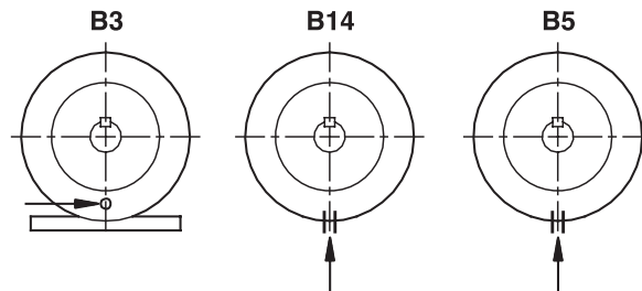
Рис. 7 Сливные отверстия
