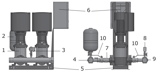
Рис. 1 Компоненты Hydro-ME
