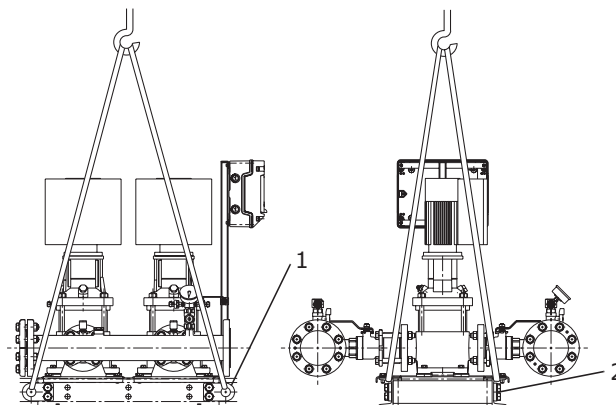
Рис. 3 Подъём установки Hydro-ME с С-образной рамой-основанием
